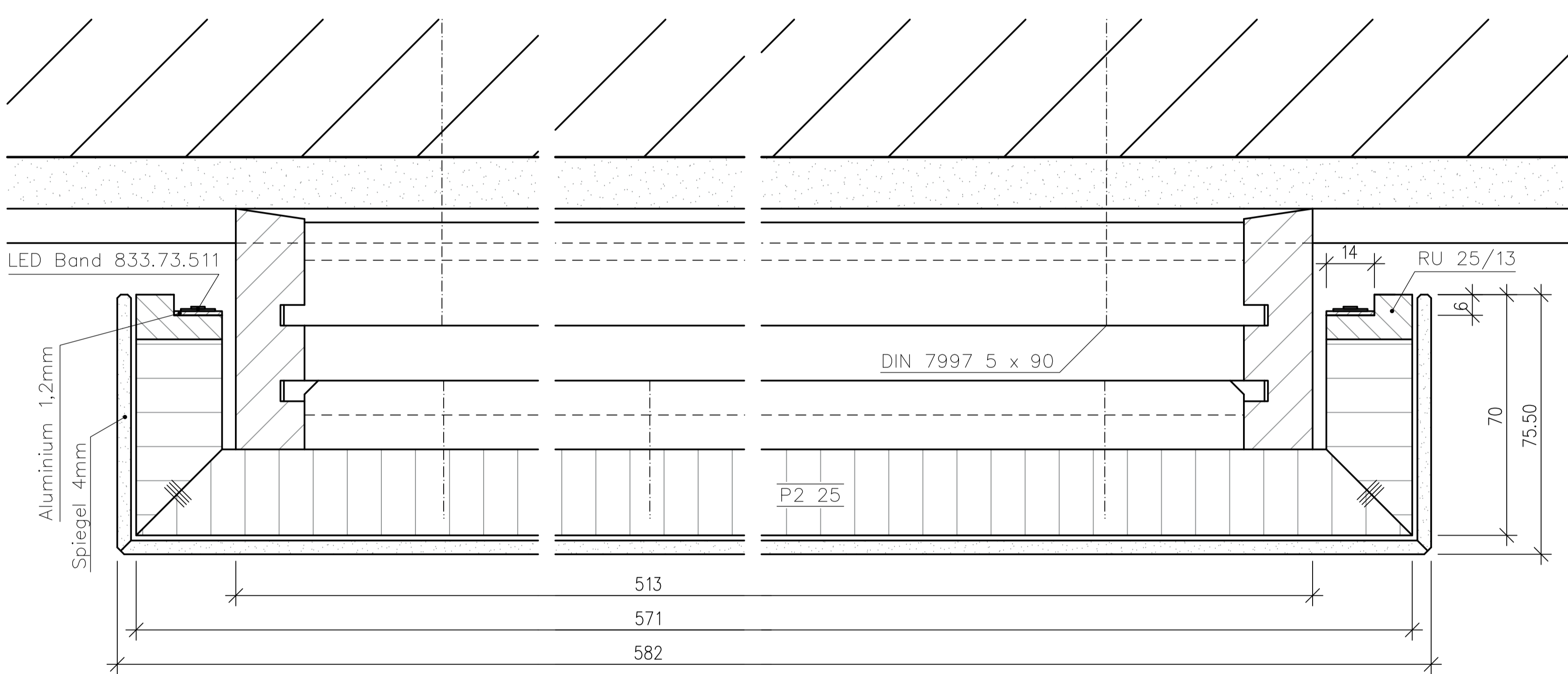
Schnitt A2 – A2
