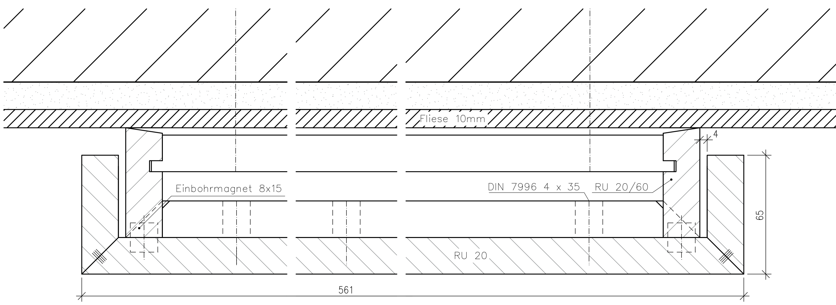
Schnitt A1 – A1
