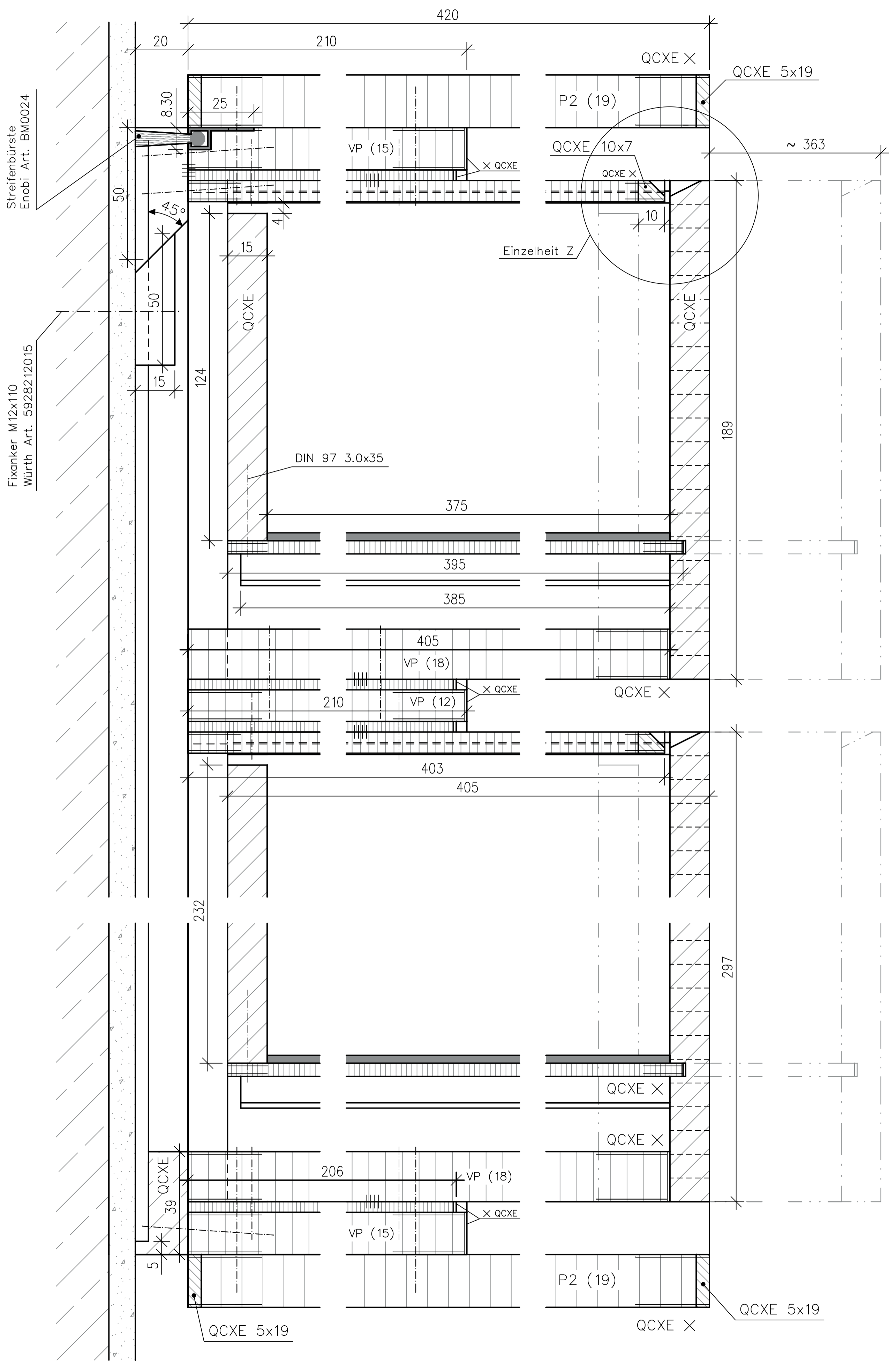
Vertikalschnitt C – C
