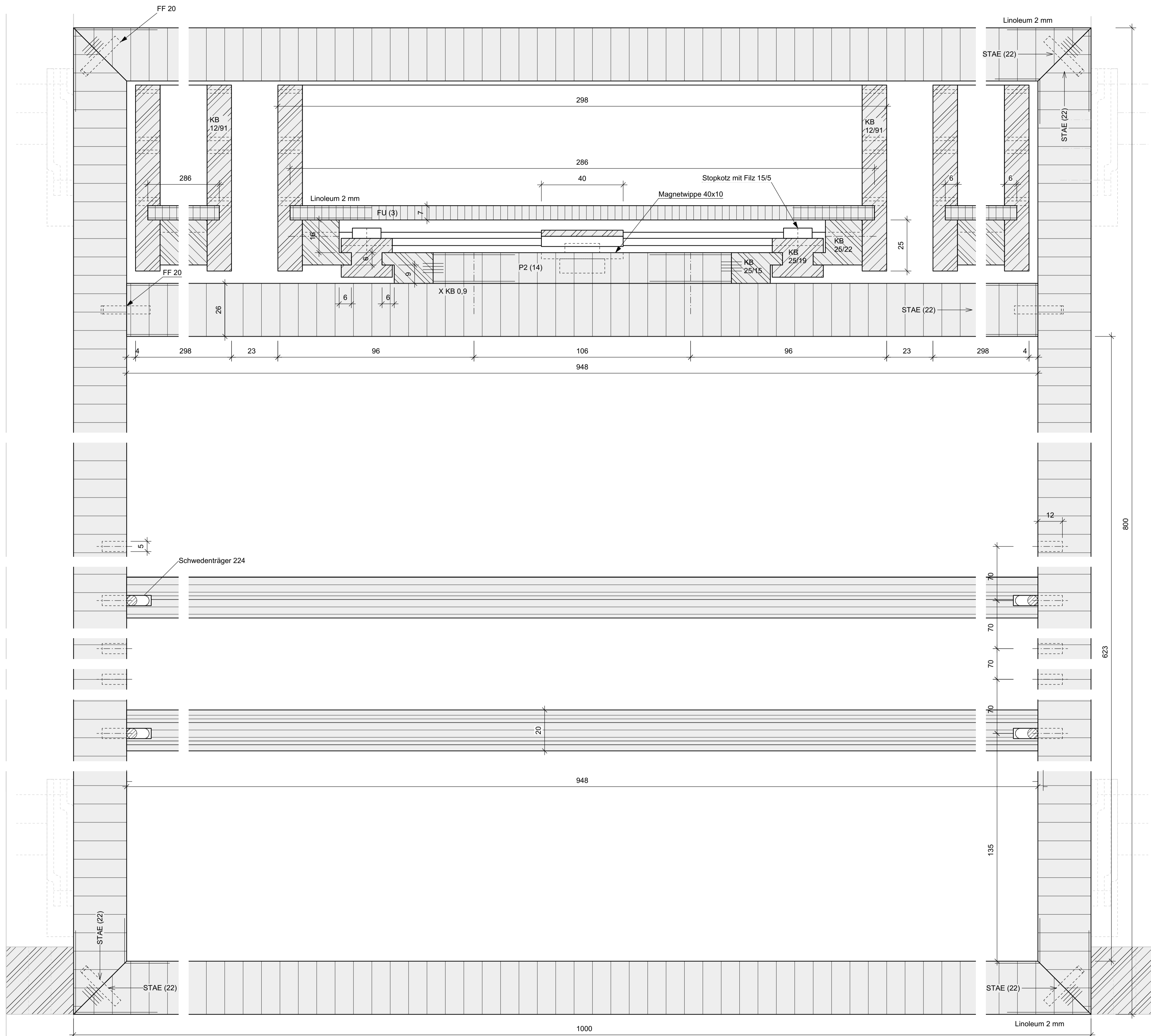
Schnitt C2-C2
