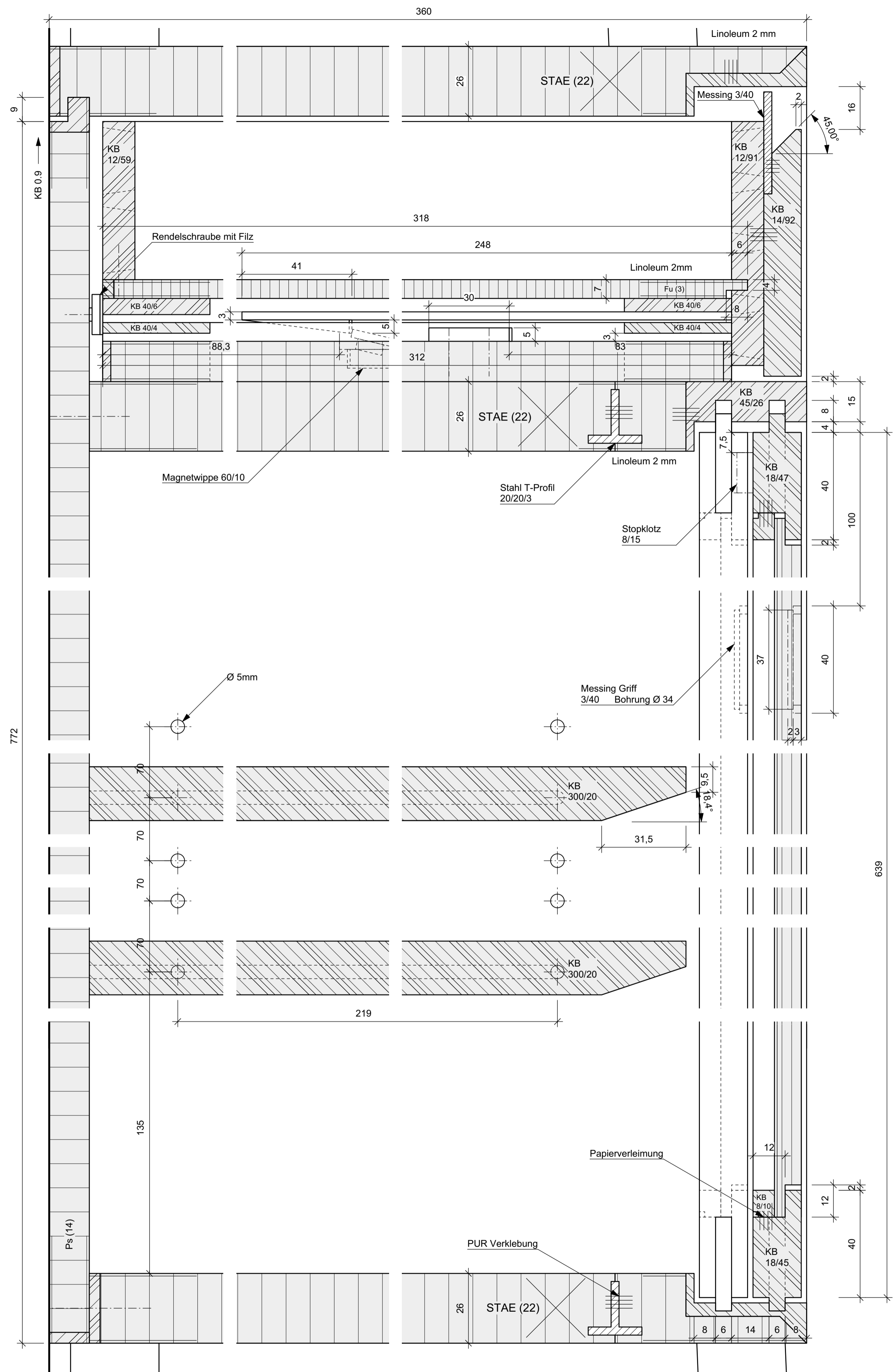
Schnitt B2-B2
